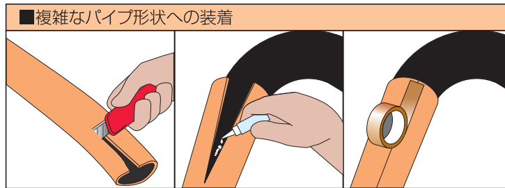
■複雑なパイプ形状への装着 ロールバーパッドを縦割りにする。パイプに巻き付け瞬間接着剤か両面テープで固定する。アセテートテープで継ぎ目を仕上げる。
