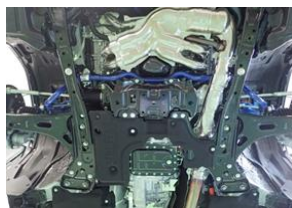
フォレスター (SLG/SL5) スタビライザー フロント
