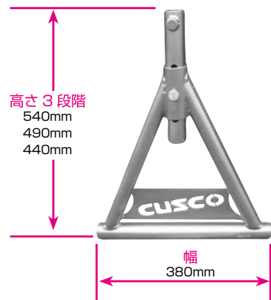
対応荷重 1.5t (左右2脚使用時)
