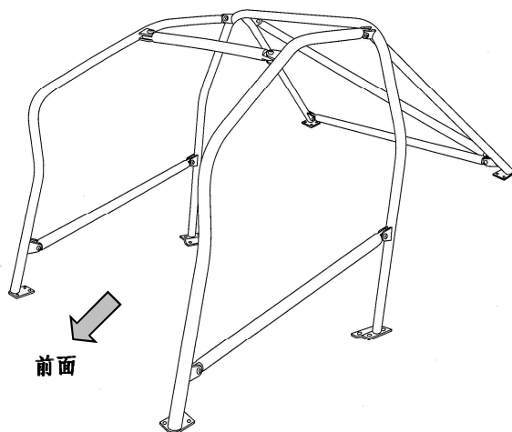
*产品样图：40ΦJ项改(*1)，10点式
