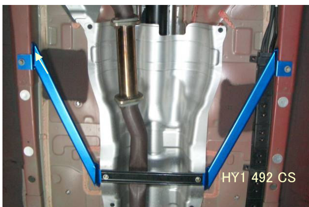
底盘加强杆 中底侧
