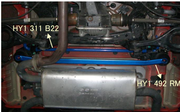
后平衡杆 后底加强件 安装图
