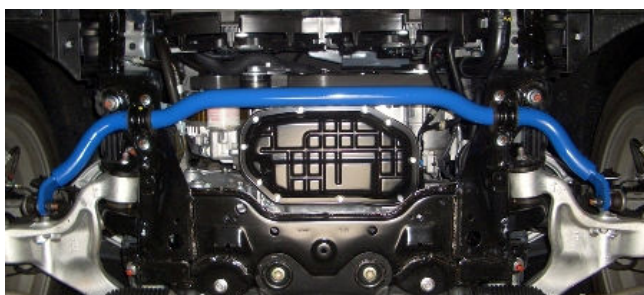
平衡杆 前 安装图
