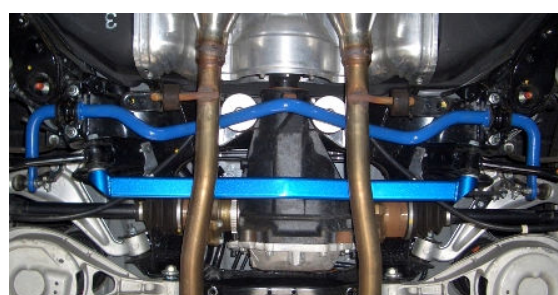
平衡杆 后/底盘加强件 后底 安装图
